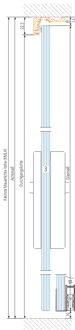
Schnitt C (Tür Raumhoch)
